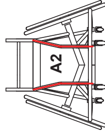
TELAIO ANTERIORE A1 con Sedile sagomato
